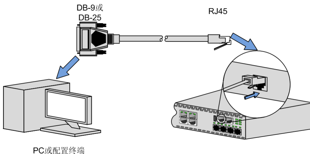
图 3-11 连接串口线
