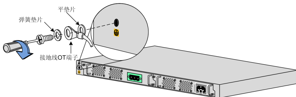
图 3-8 连接接地线缆
