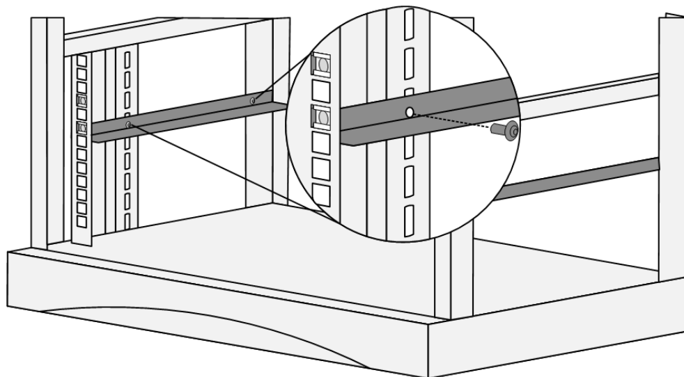
图 3-3 安装滑道
