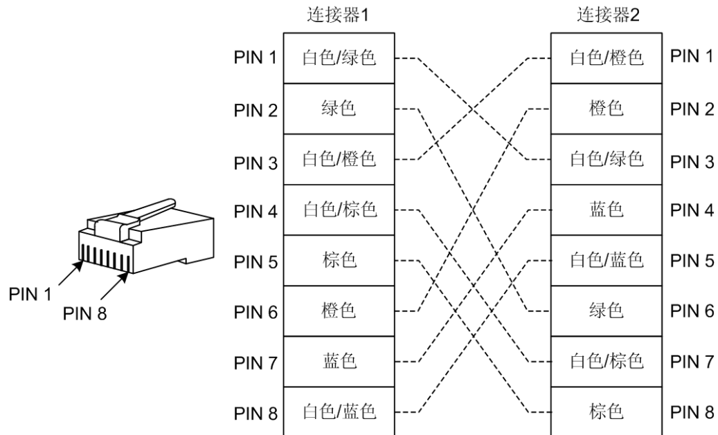
图 5-6 1000Mbit/s 交叉网线接线图
