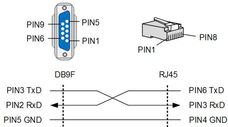
图 5-13 接线关系示意图
