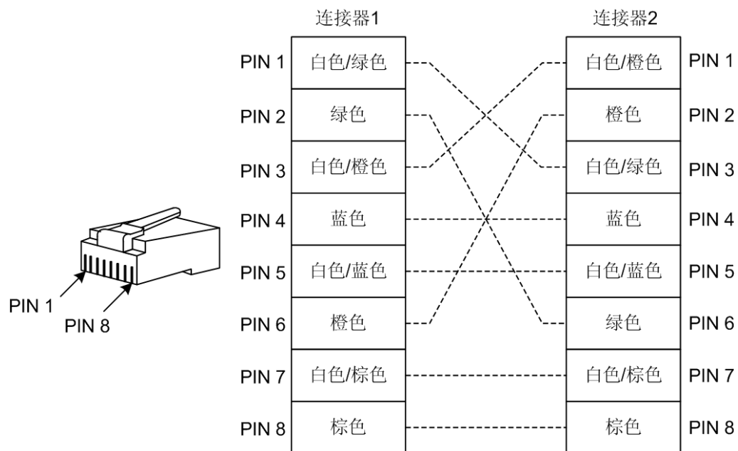
图 5-5 100Mbit/s 交叉网线接线图
