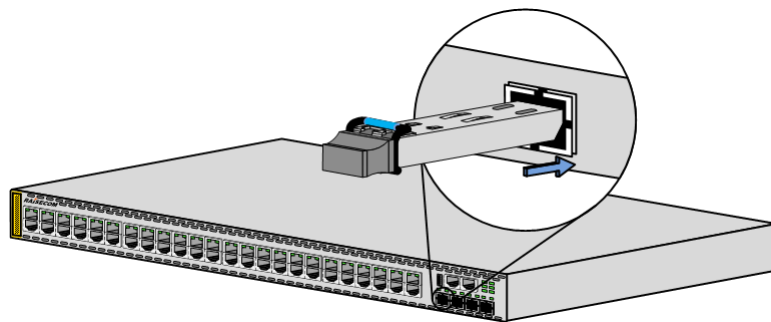
图 3-5 插入 SFP 光模块
