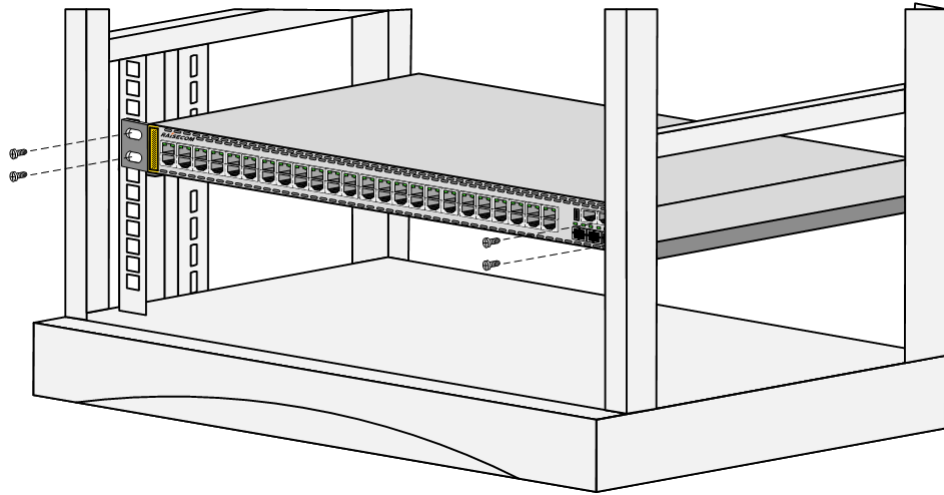
图 3-4 水平安装设备到机柜
