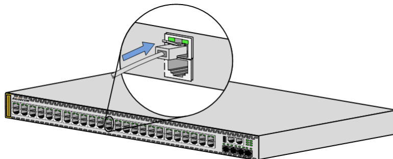
图 3-7 连接以太网线
