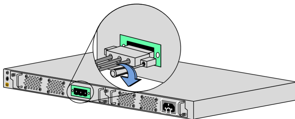
图 3-9 连接直流线缆
