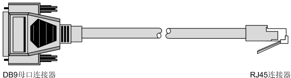
图 5-12 RJ45 类型串口线示意图
