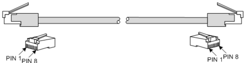
图 5-2 网线示意图
