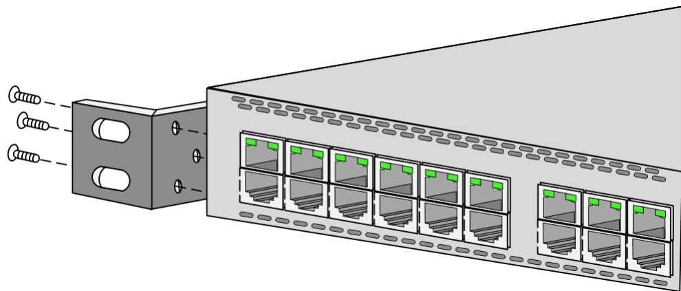
图3-1 安装挂耳
