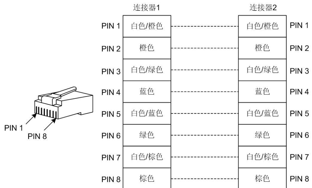
图 5-4 10/100/1000M 直通网线接线图
