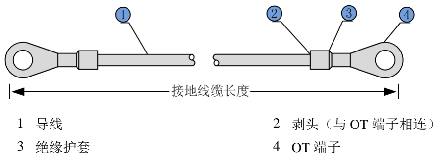
图 5-7 接地线缆示意图
